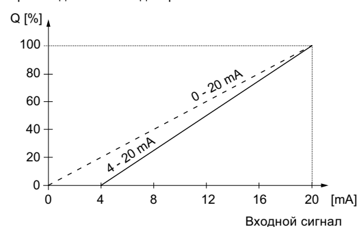
Рис. 10 Управление 0/4-20 мА
