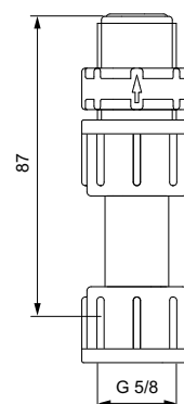
Рис. 44 Нагнетательный клапан
