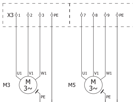
Дренажный насос
