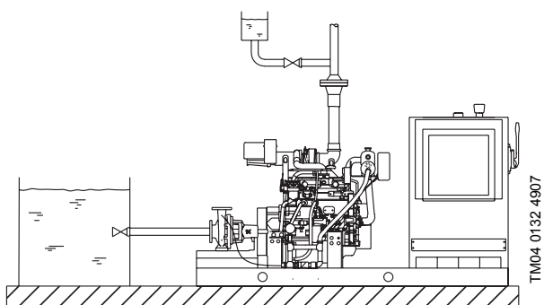
Рис. 24 Схематическое изображение открытой системы с насосом NKF
