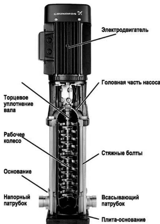
Рис. 4 Жockey-насос
