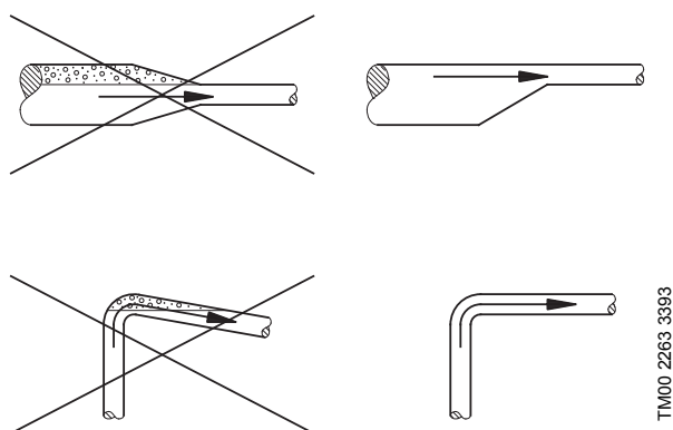
Рис. 28 Установка трубопроводов
