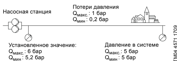
Рис. 29 С режимом пропорционального регулирования напора
