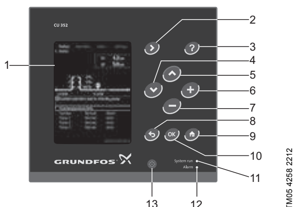
Рис. 9 Панель управления CU 352
