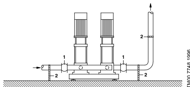
Рис. 8 Крепление трубопровода
