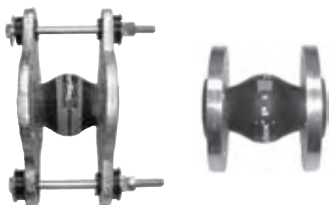
Рис. 34 Вибровставки с резиновыми прокладками без ограничительных стяжек и с ними
