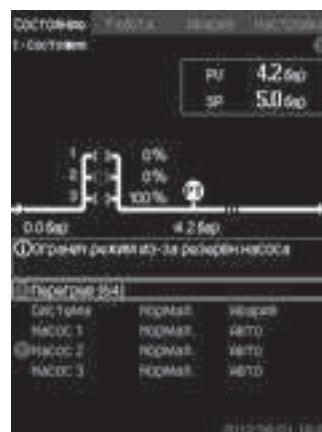
Рис. 10 Меню "Состояние"
