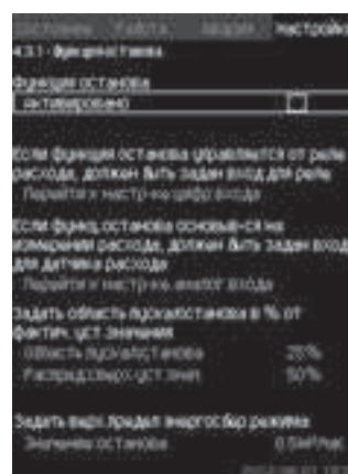
Рис. 20 Функция останова
