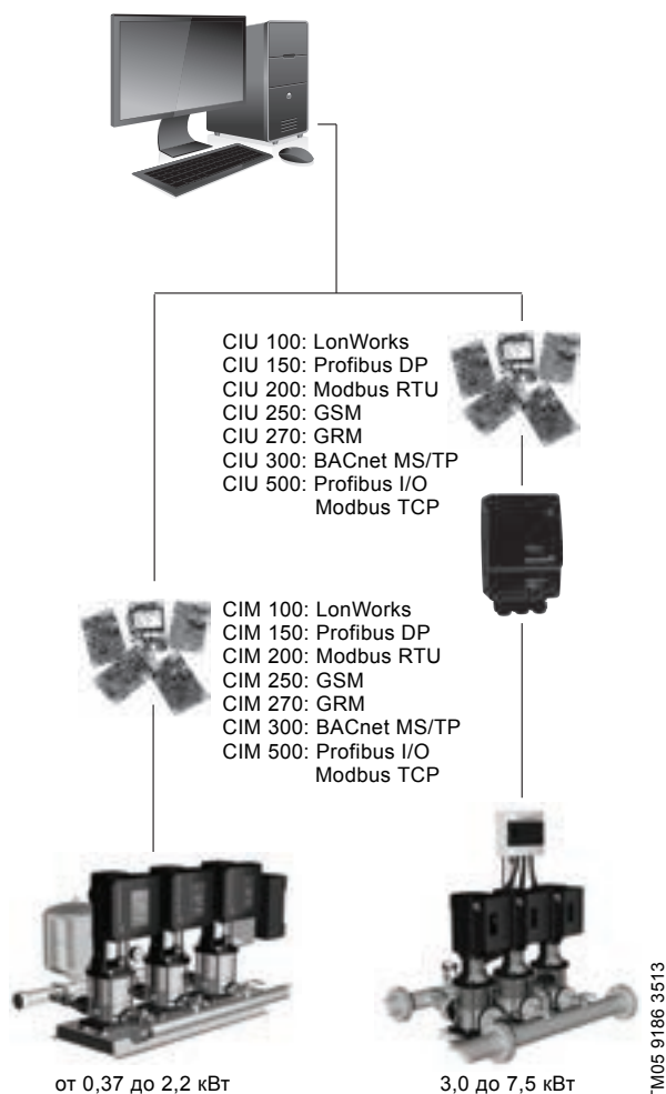
Рис. 13 Структура системы управления внутридомовыми коммуникациями
