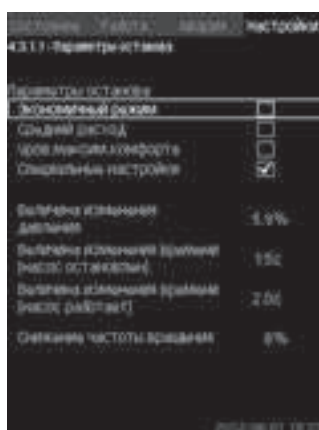
Рис. 22 Параметры остановки
