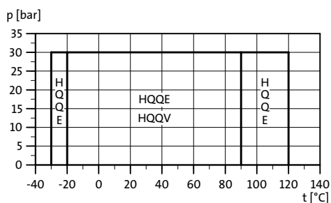
Рис. 14 Область эксплуатации стандартных уплотнений вала
