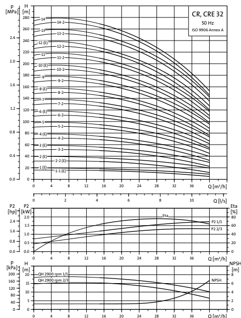
Рис. 15 График производительности
