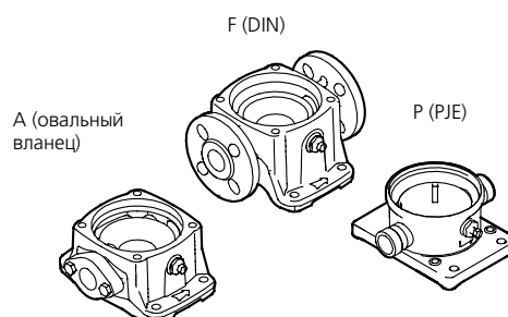
Рис. 22 Соединения насоса
