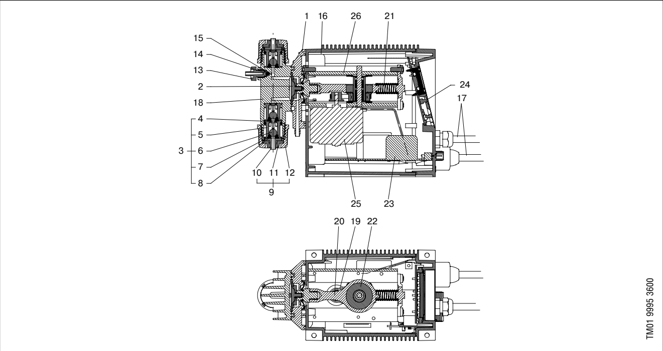
Чертеж в разрезе, DMS
