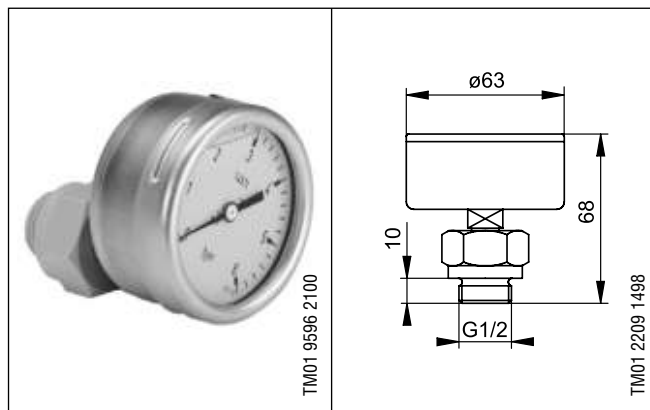
Манометр
