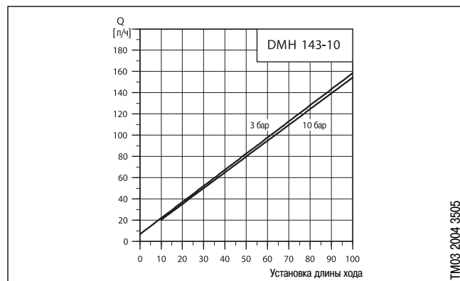
DMH 143-10
