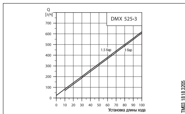
DMX 525-3
