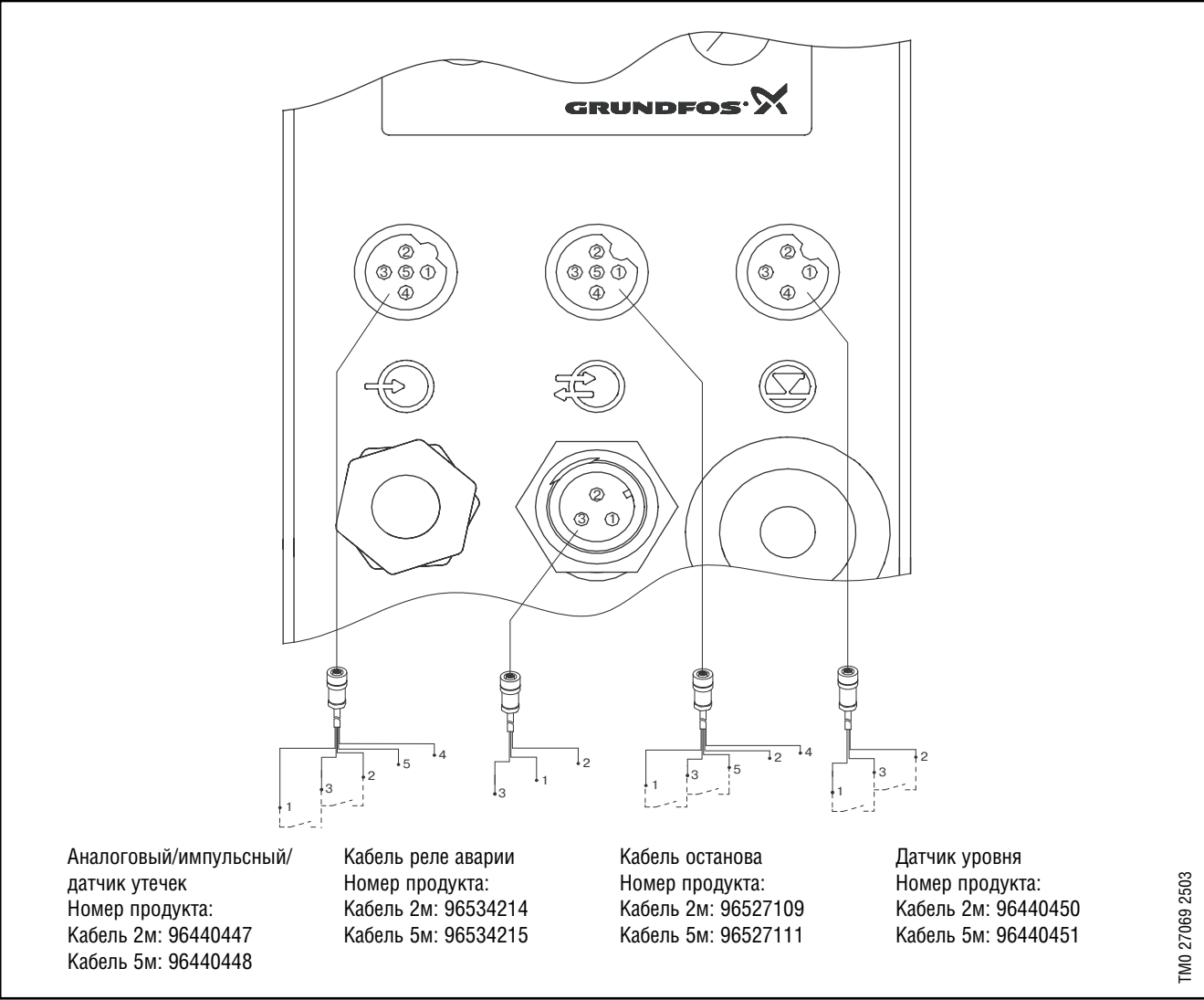
Кабель 1: Вход для аналогового, импульсного сигналов и сигнала от датчика разрыва диафрагмы
