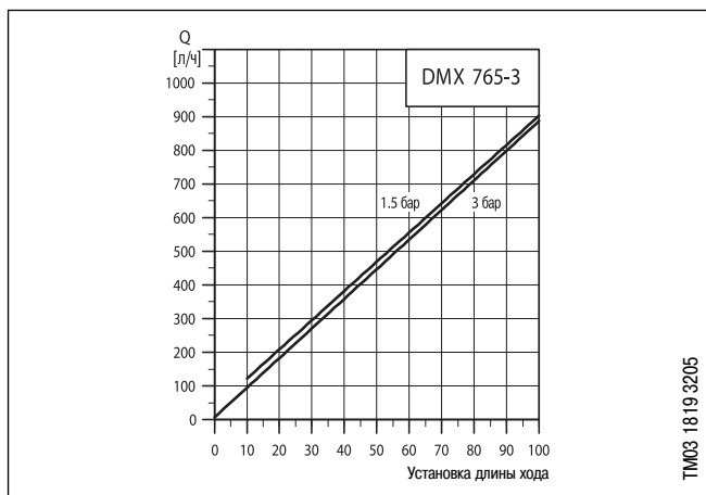
DMX 765-3
