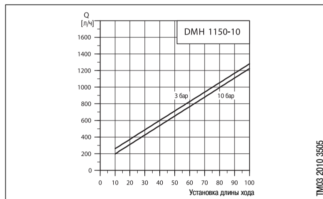
DMH 1150-10
