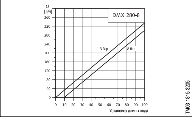
DMX 280-8
